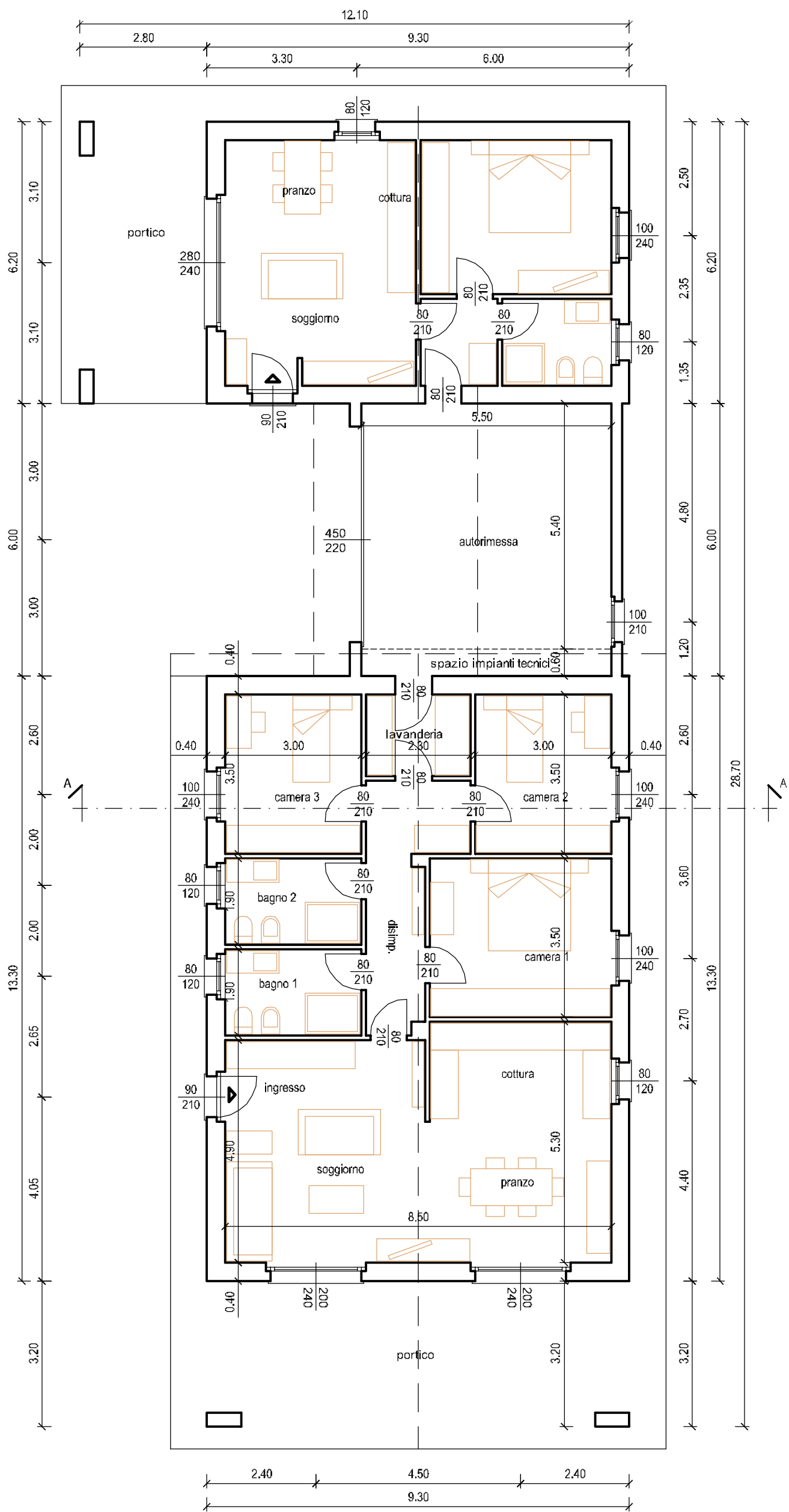
PIANTA PIANO TERRA
